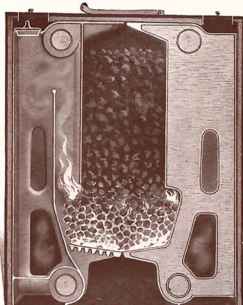
Querschnitt mit Zug der Gase
